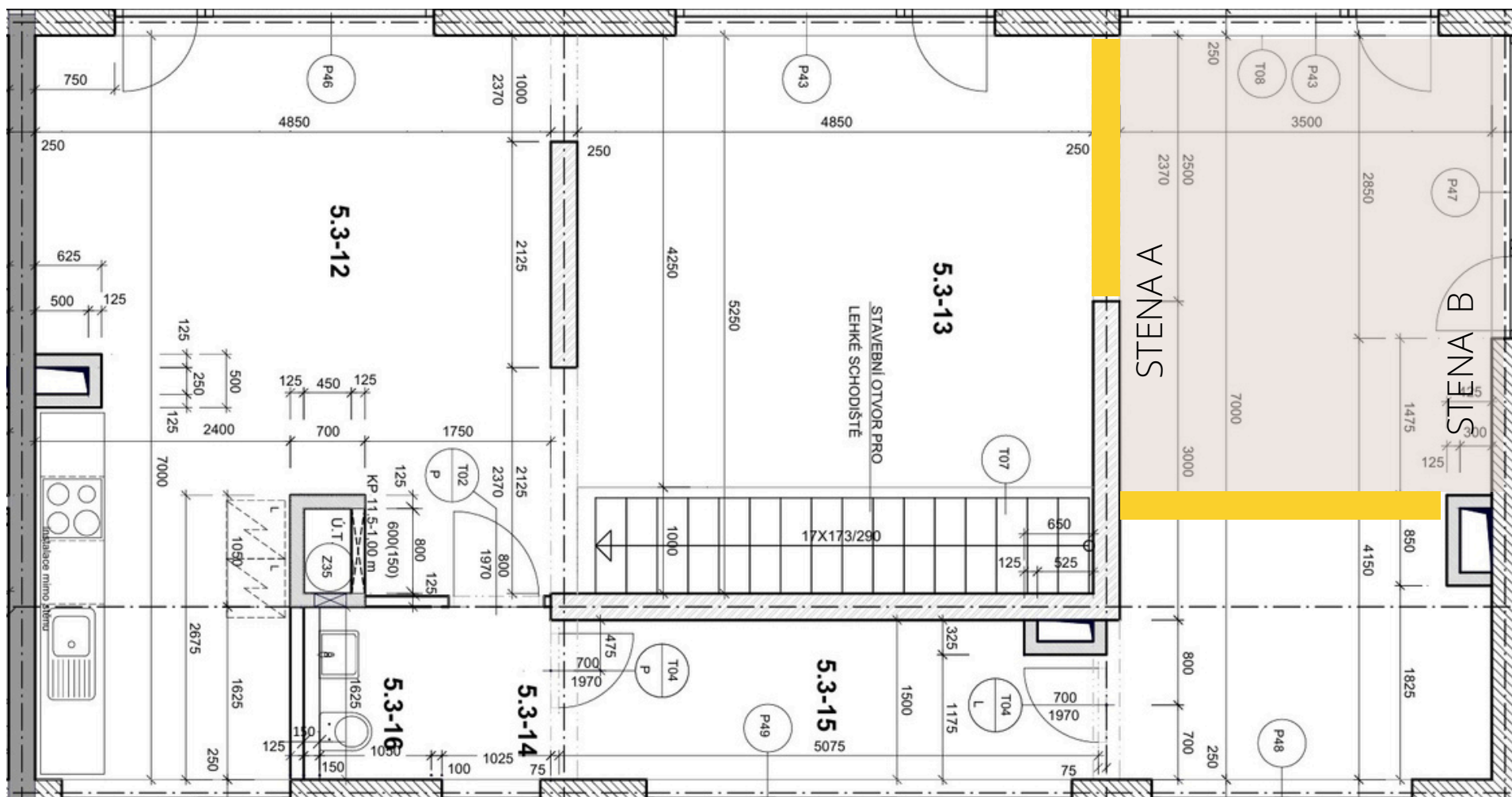
LOŽNICE - 5.3.-13
