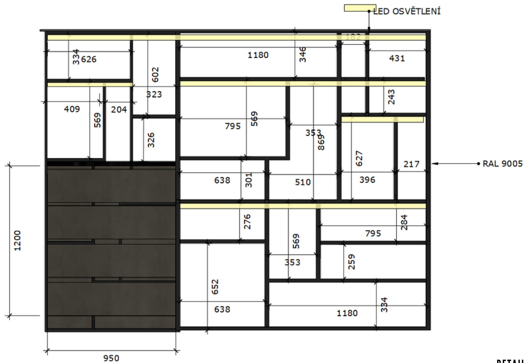
DETAIL SKŘÍNĚ
