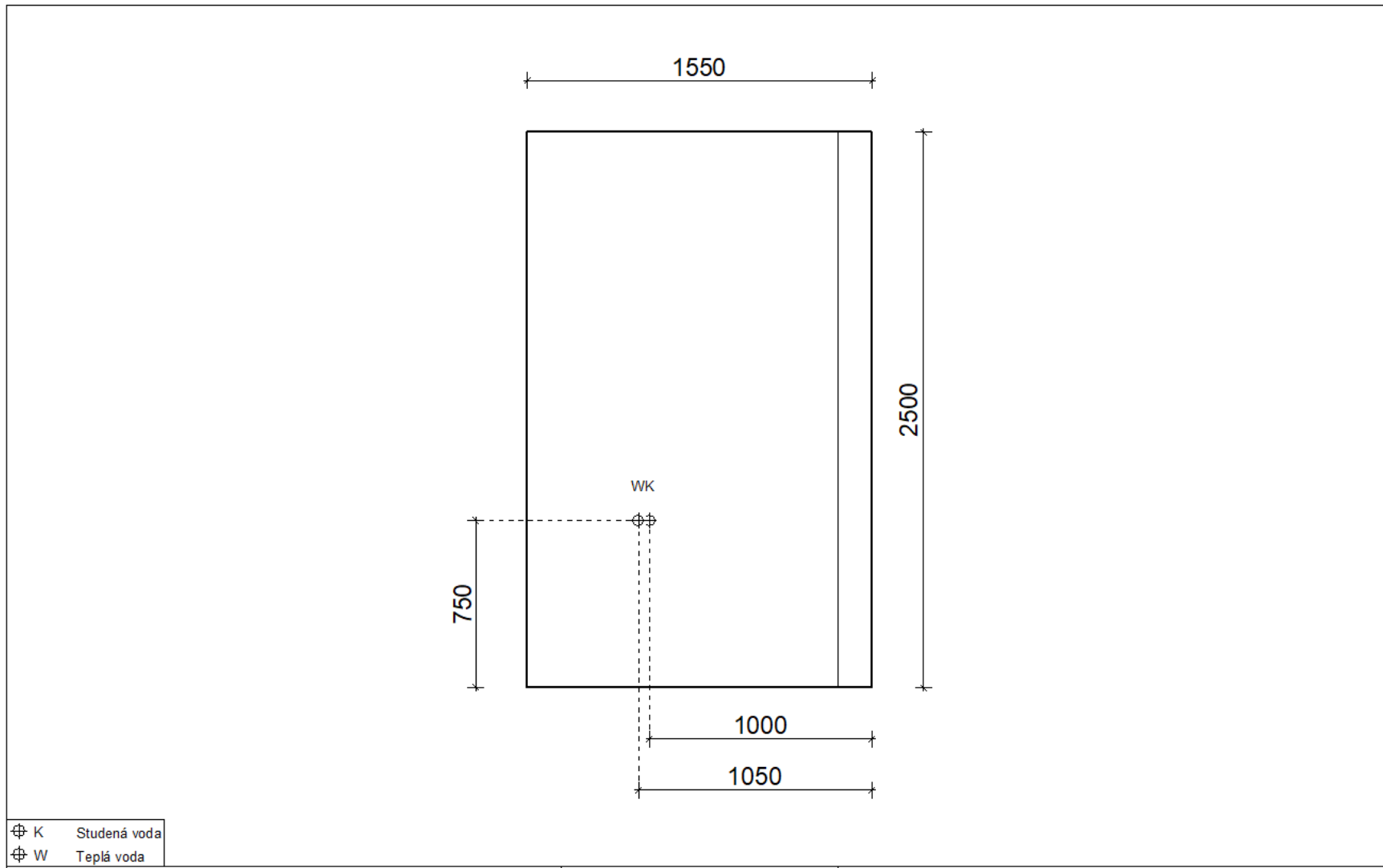
Koupelna 2.05 –stěna - 6
