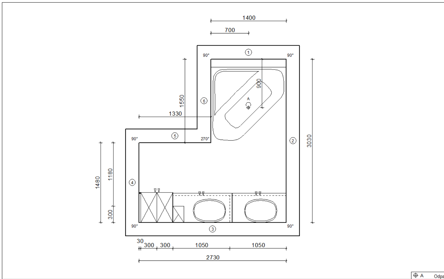
Koupelna 2.05 – půdorys
